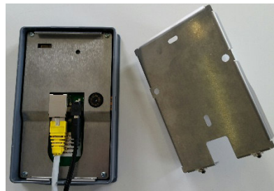
Figure 10b : Raccordement du câble d'alimentation et du câble LAN au dos de l'appareil
