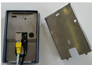
Figures 9b: Raccord de la prise de courant et du câble LAN au dos de l'appareil
